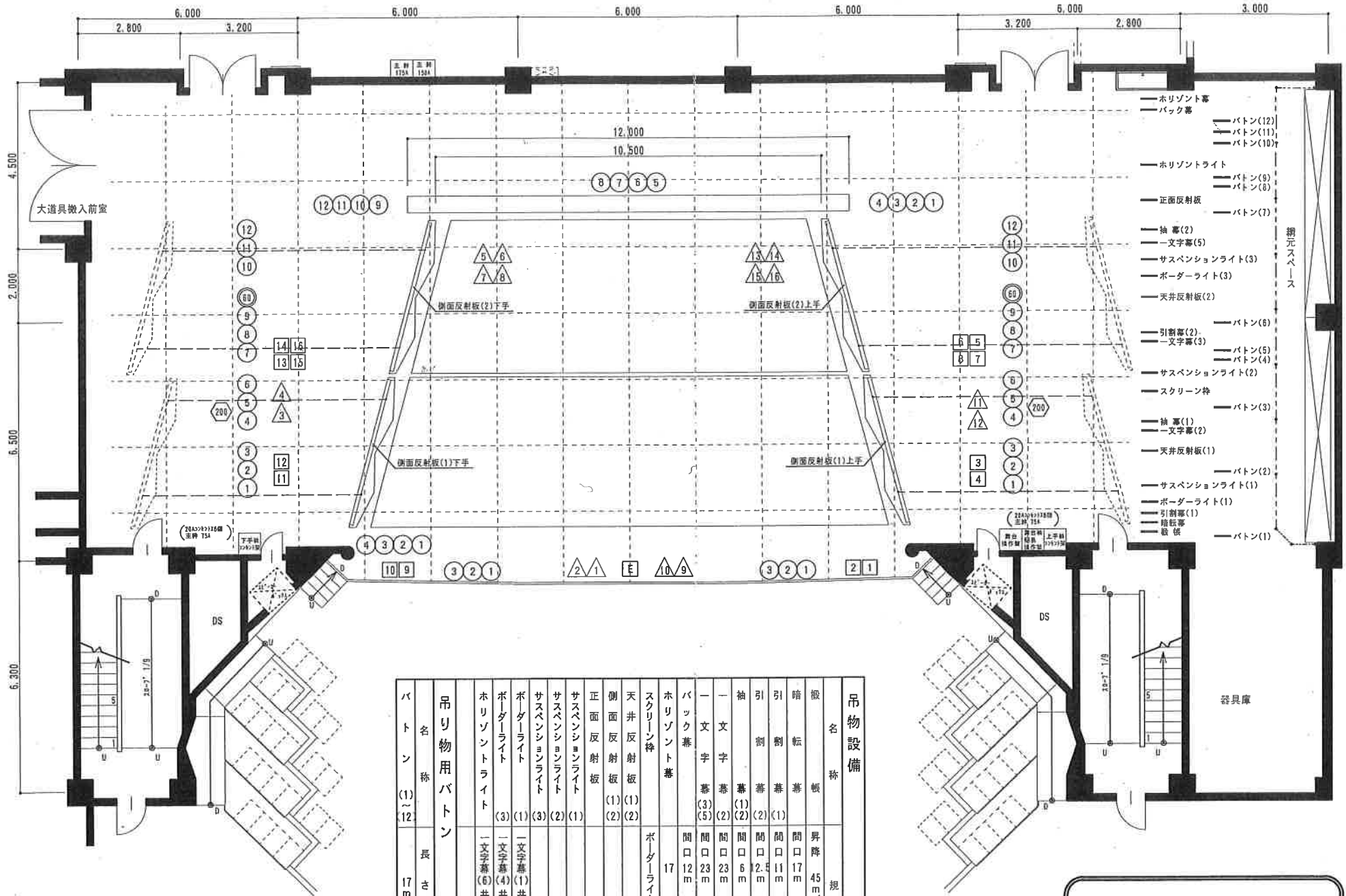
松前総合文化センター 舞台平面図 縮尺 1/100
